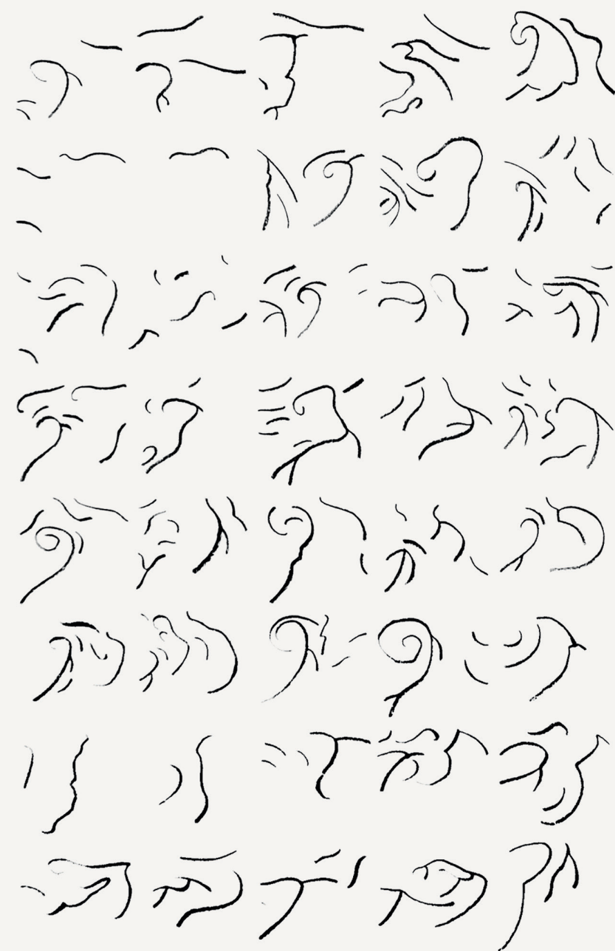
40 Variations des fronts froids et chauds Sur l'Europe, du 29 juin au 20 août 2009
